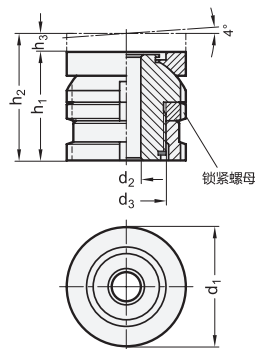
垫圈 GN 6339
